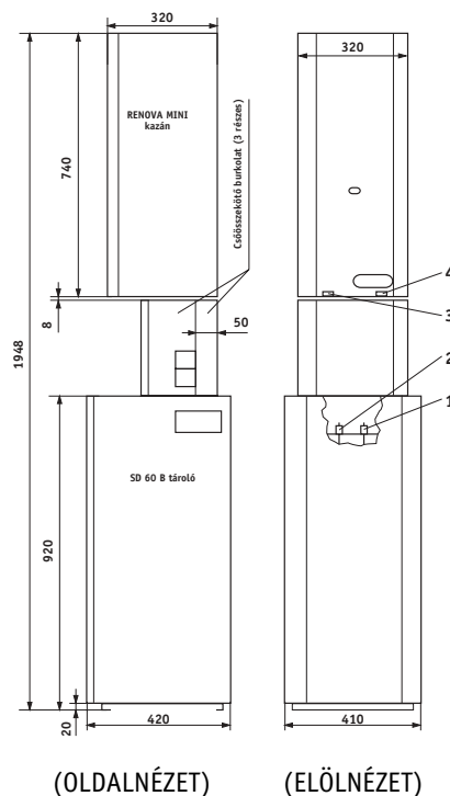
10. ábra RENOV MINI hőközpont fő méretek kazán alá telepített tároló változathoz
