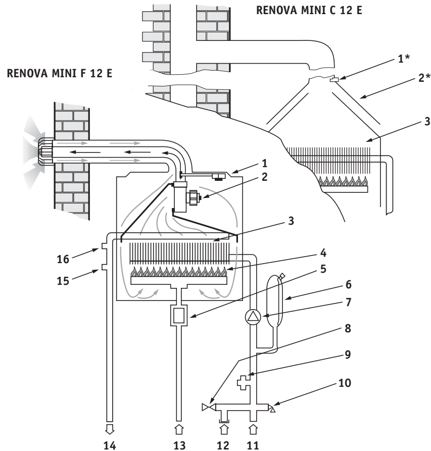
3. ábra A RENOVA MINI felépítése
