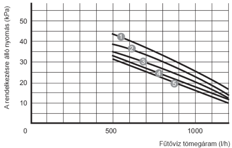
7. ábra A RENOVA STAR kazánok szivattyújának jelleggörbéje
