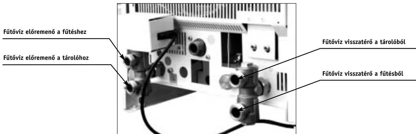
8. ábra – A csőösszekötő készlet csatlakoztatása a kazánra (alulnézetben)
