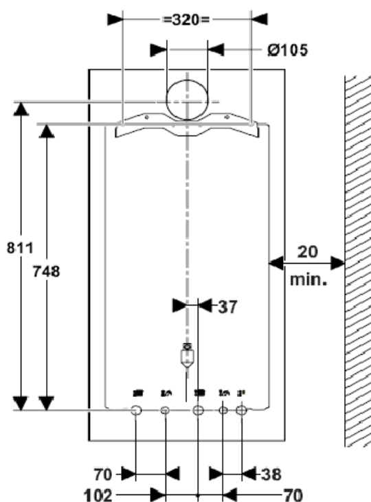
12. ábra A RENOVA STAR kazán elhelyezése
