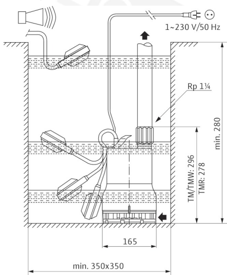
Méretrajz Wilo-Drain TM/TMW/TMR 32/8
