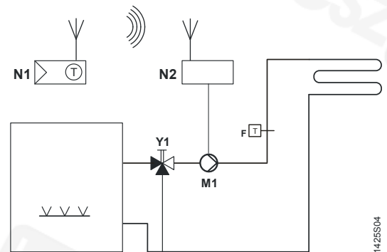
Vezeték nélküli szobatermosztát vevőegységgel, hidraulikus padlófűtési rendszer direkt szabályozásával
