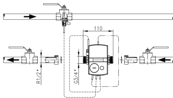
Beépítés érzékelő fogadó golyóscsap alkalmazásával
