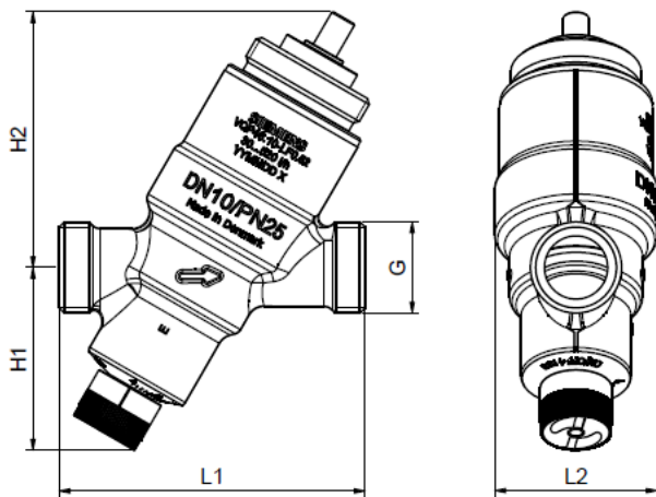
VQP46..
