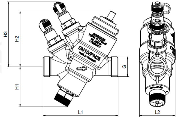
VQP46..Q
