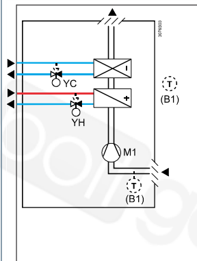
4-pipe fan coil unit
