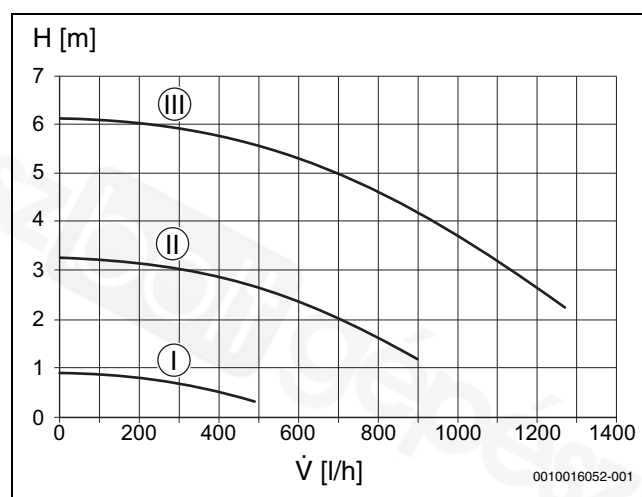
44. ábra A fűtési szivattyú jelleggörbéje (állandó fordulatszám)
