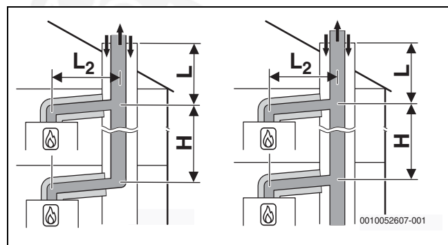
25. ábra Több készülék bekötése C (14)3x szerint közös, merev füstgázvezetéssel és koncentrikus levegő-/füstgázvezetés a felállítási helyiségben
